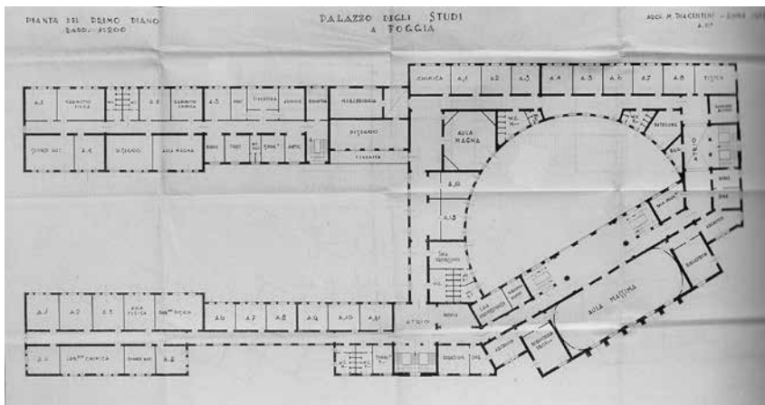
M. Piacentini, Foggia – Palazzo degli studi, pianta primo piano, 1928
